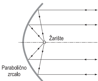
ZRCALO, PARABOLIČNO, shema refleksije svjetlosti
